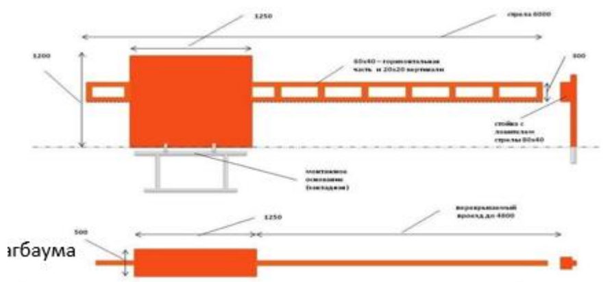
Рис. 2. Внешний вид шлагбаума.
